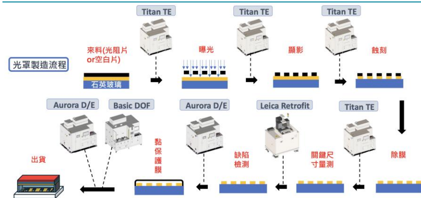
圖表 2：光罩檢測機應用
