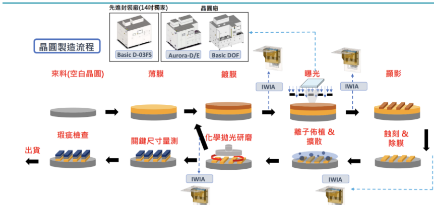
圖表 3：晶圓檢測機應用
